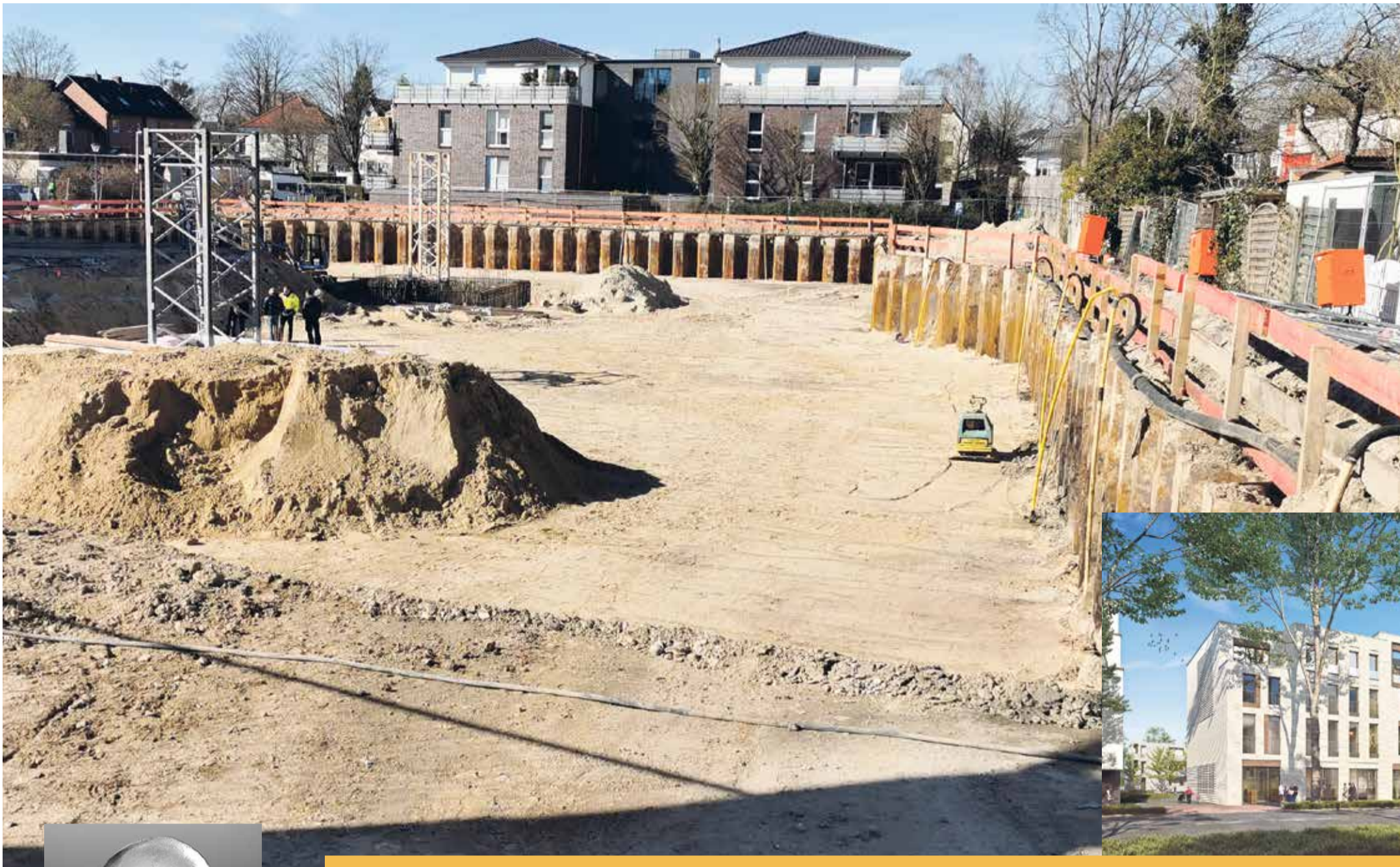
Ein Blick in die komplizierte Baugrube: Die Spundwand steht.
